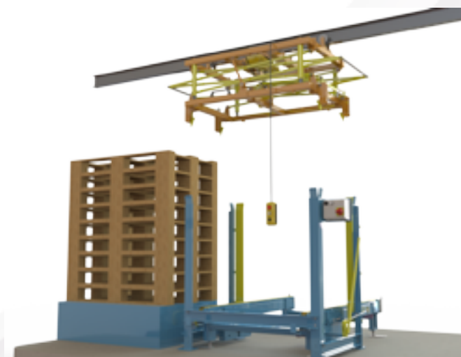
Dépileur de palettes aérien manuel
